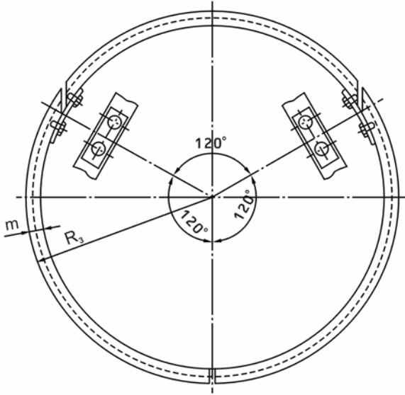
■套管用中間圈
