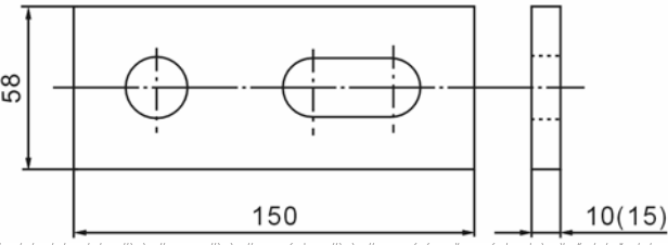
■中間圈用卡具(CNS 2473-SS 400 或尼龍 6)
