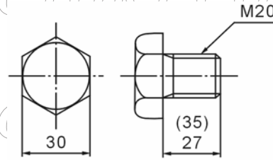
■中間圈用卡具用螺栓
